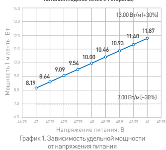
Зависимость мощности 1 м ленты от напряжения питания (подключение с 1 стороны)
